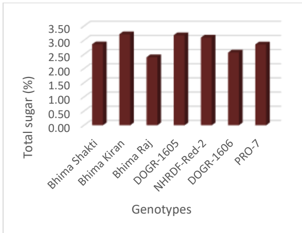
Fig. 5. Genotypes TS
